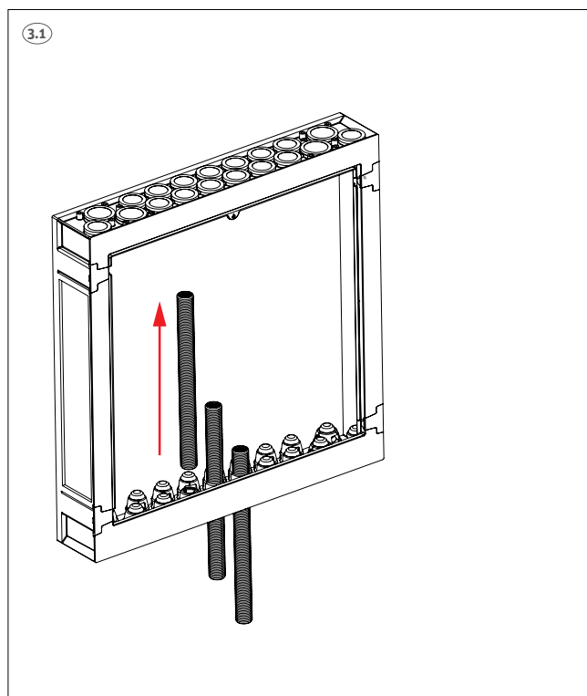
3.1. Demonter varerør fra fordelerskap.
