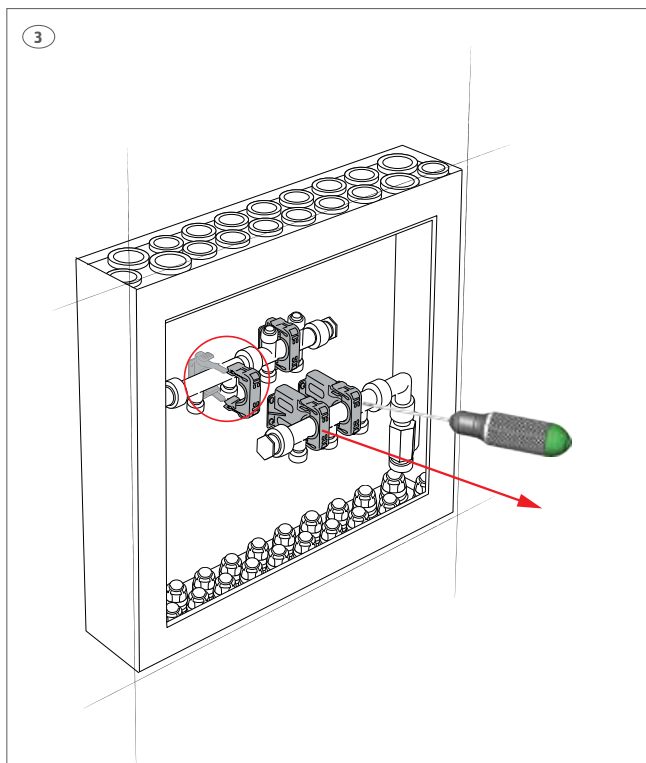
3. Demonter fordeler fra fordelerfestene, la fordelerfestene ligge i bunnen av skapet.
