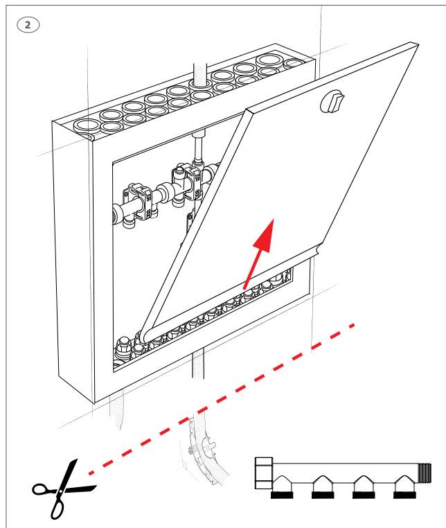
2. Klipp av rør eller demonter rør fra fordeler.
